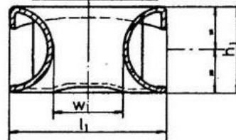
SECCION A-A
